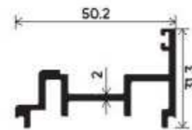
Door Adaptor Section Number : V-5208 Weight (kg/mt) : 0.669
