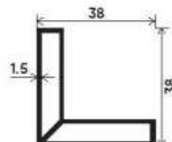
38 x 38 Angle Section Number : V-2740 Weight (kg/12') : 2.038
