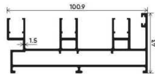
Premium Type Section Number : V-2504 Weight (kg/mt) : 1.676
