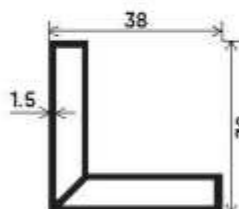
38 x 38 Angle Section Number : V-2740 Weight (kg/12') : 2.038
