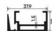
Slim Interlock DGU Section Number : V-3117 Weight (kg/m) : 0.683
