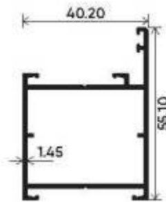
Door Frame Section Number : V-4026 Weight (kg/mt) : 0.754
