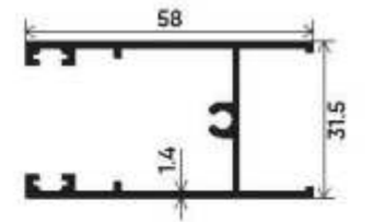
Top & Bottom Shutter Section Number : V-3512-1 Weight (kg/mt) : 0.700
