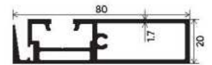
Box Reinforcement Interlock S. G. Section Number : V-3122 Weight (kg/m) : 1.202
