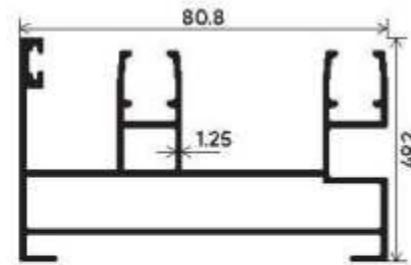
Premium Type Section Number : V-3552 Weight (kg/mt) : 1.230
