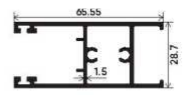
Top & Bottom DGU Shutter Section Number : V-3116 Weight (kg/m) : 1.079
