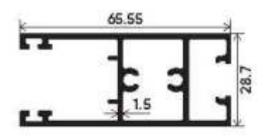
Top & Bottom S. G. Shutter Section Number : V-3112 Weight (kg/m) : 1.079
