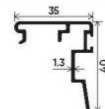
Universal Clip Section Number : V-2521 Weight (kg/mt) : 0.393
