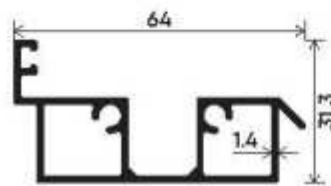
Bottom Guide Section Number : V-5203 Weight (kg/mt) : 0.902
