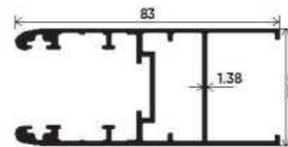
DGU Shutter Section Number : V-3712 Weight (kg/mt) : 1.230
