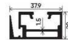
Slim Interlock S. G. Section Number : V-3121 Weight (kg/m) : 0.683
